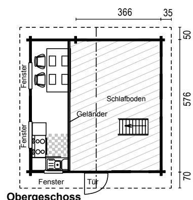
Obergeschoss
