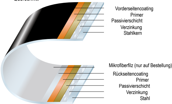
Querschnitt
